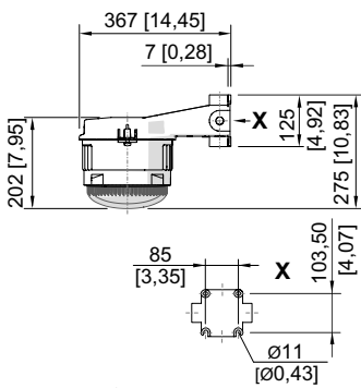
Montage au plafond sans panier de protection
