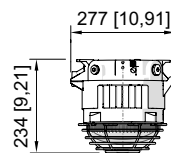
Montage en suspension avec vis à œil
